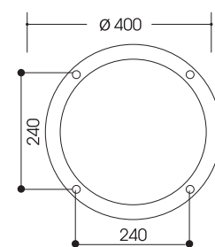
Đế cột Base plate
