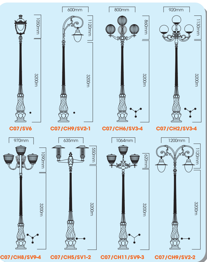
Chiếu sáng Đèn Quốc Tổ Lạc Long Quân Khu di tích lịch sử Đèn Hùng - Phú Thọ
